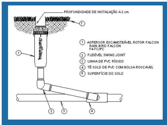
Figura 5: Detalhes da correta instalação de um aspersor de rotor com swing joint
