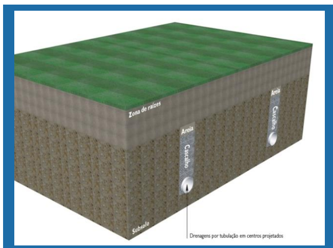
Figura 2: Perfil de um campo com tubulações de drenagem em solo natural
