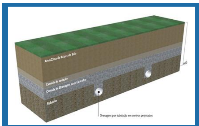
Figura 3: Perfil de um campo com camada arenosa sobre colchão drenante de brita
